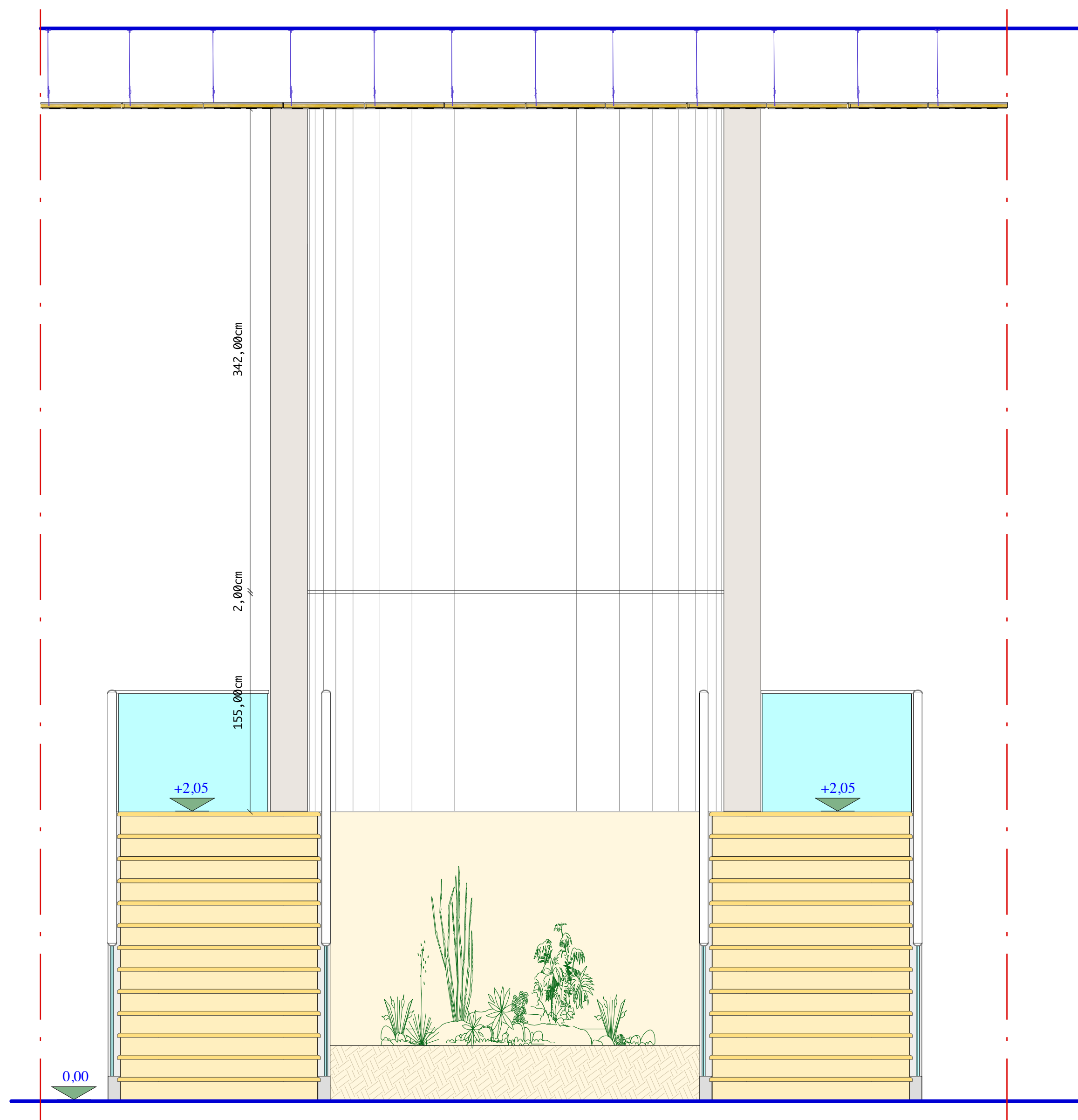
VISTA FRONTALE
